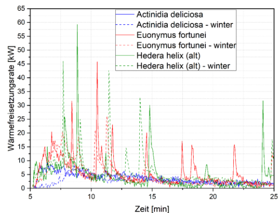
Abbildung 3: Vergleich der Wärmefreisetzungsrate von Actinidia deliciosa, Euonymus fortunei und Hedera helix im Sommer und Winter
